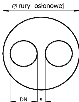
rura preizolowana
